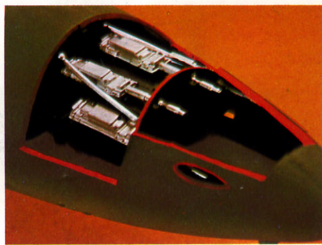
Nel muso del Me 262 vi sono i dettagli del cannone Mk 108 da 4-30mm. completo degli scivoli per le munizioni.
